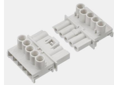
AC 164 BU/5 dişi jak AC 164 ST/5 erkek jak
