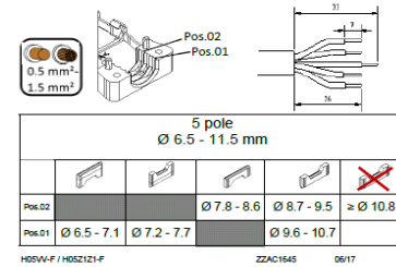
AC 164 BUF/5 kapaklı dişi AC 164 STF/5 kapaklı erkek
