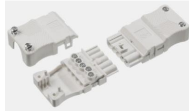
AC 164 BUF/5 kapaklı dişi AC 164 STF/5 kapaklı erkek
