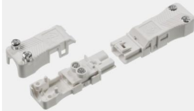
AC 164 BUF/2 kapaklı dişi AC 164 STF/2 kapaklı erkek
