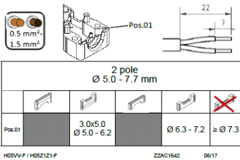
AC 164 BUF/2 kapaklı dişi AC 164 STF/2 kapaklı erkek
